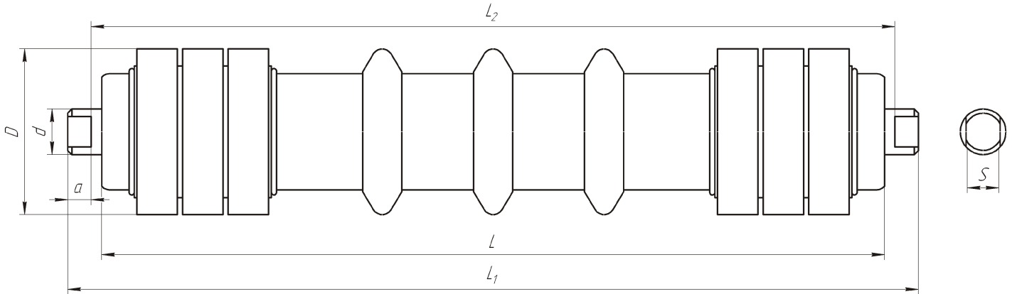
Bild 1 Scheibenrolle
