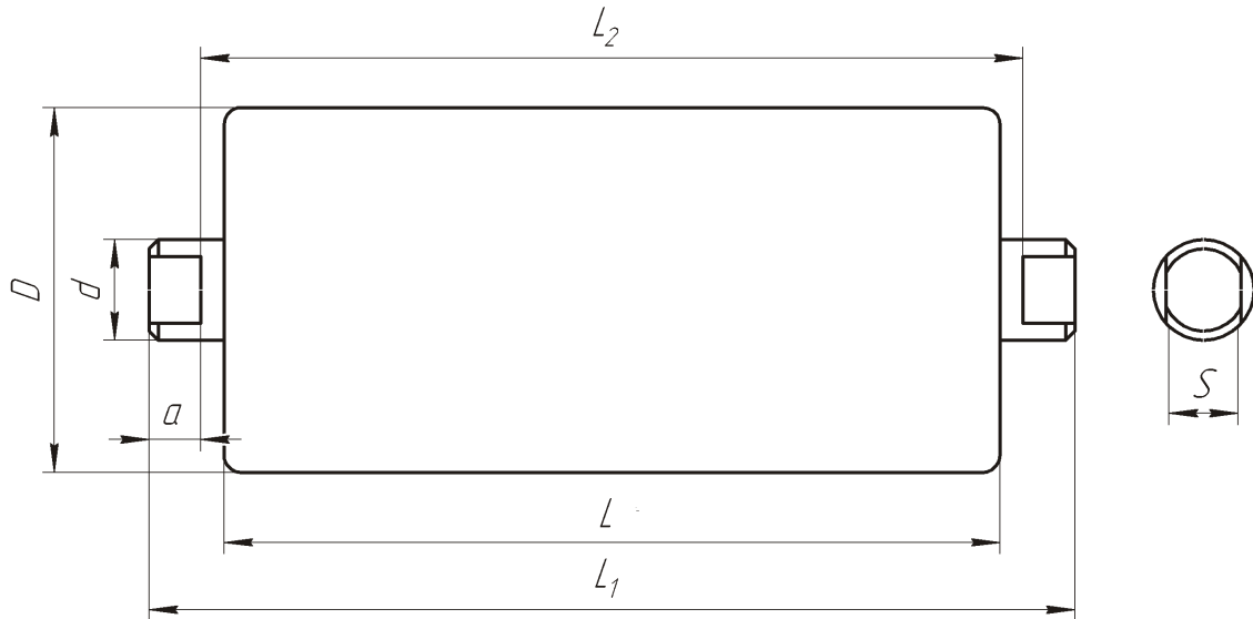
Bild 2 Blindabflachung
