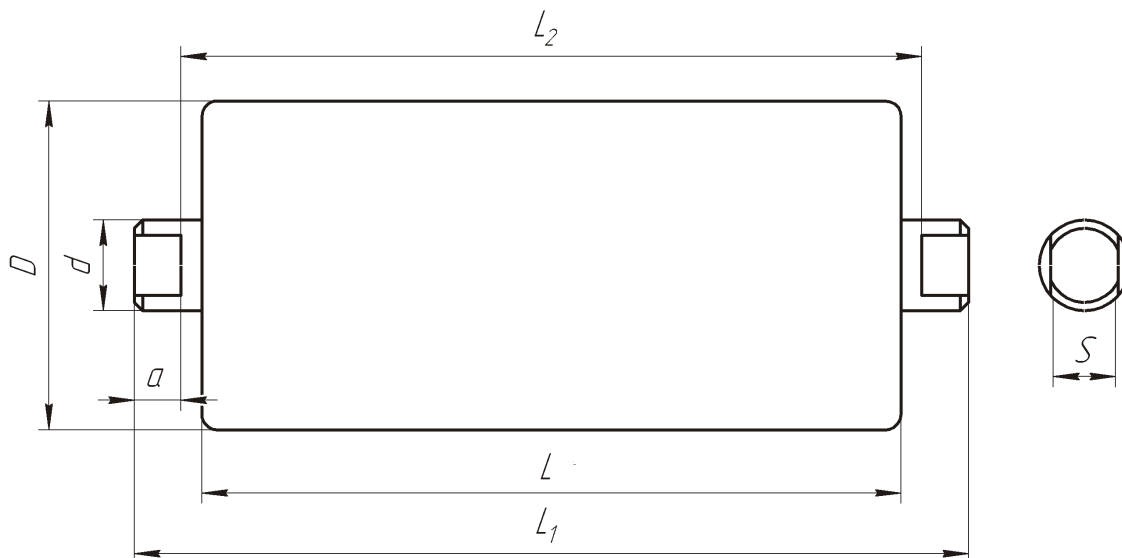
Рис.2 с глухой лыской
